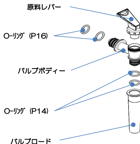
＜原料タンク弁の構成＞
